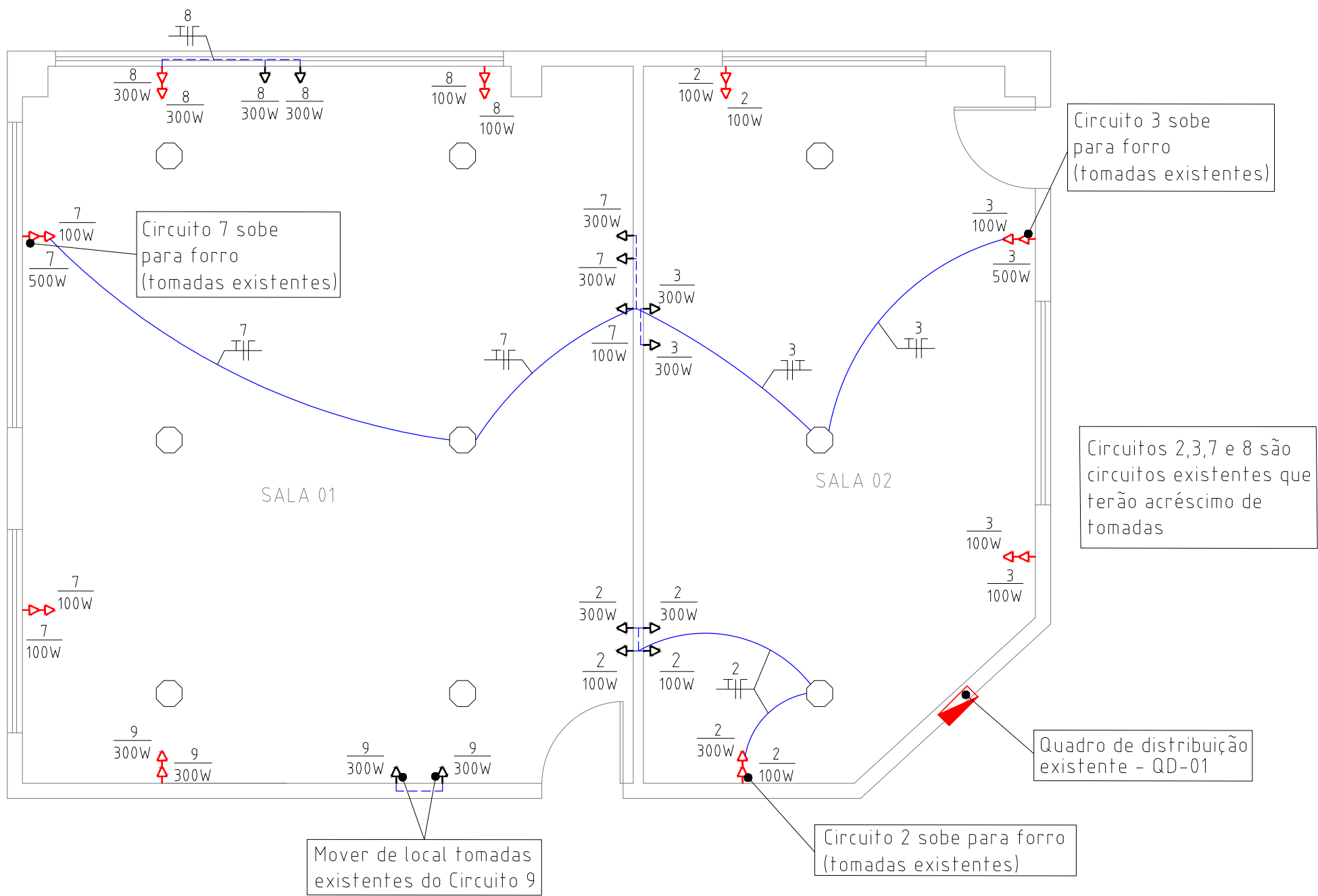
PLANTA BAIXA – TOMADAS ESC. 1:50
