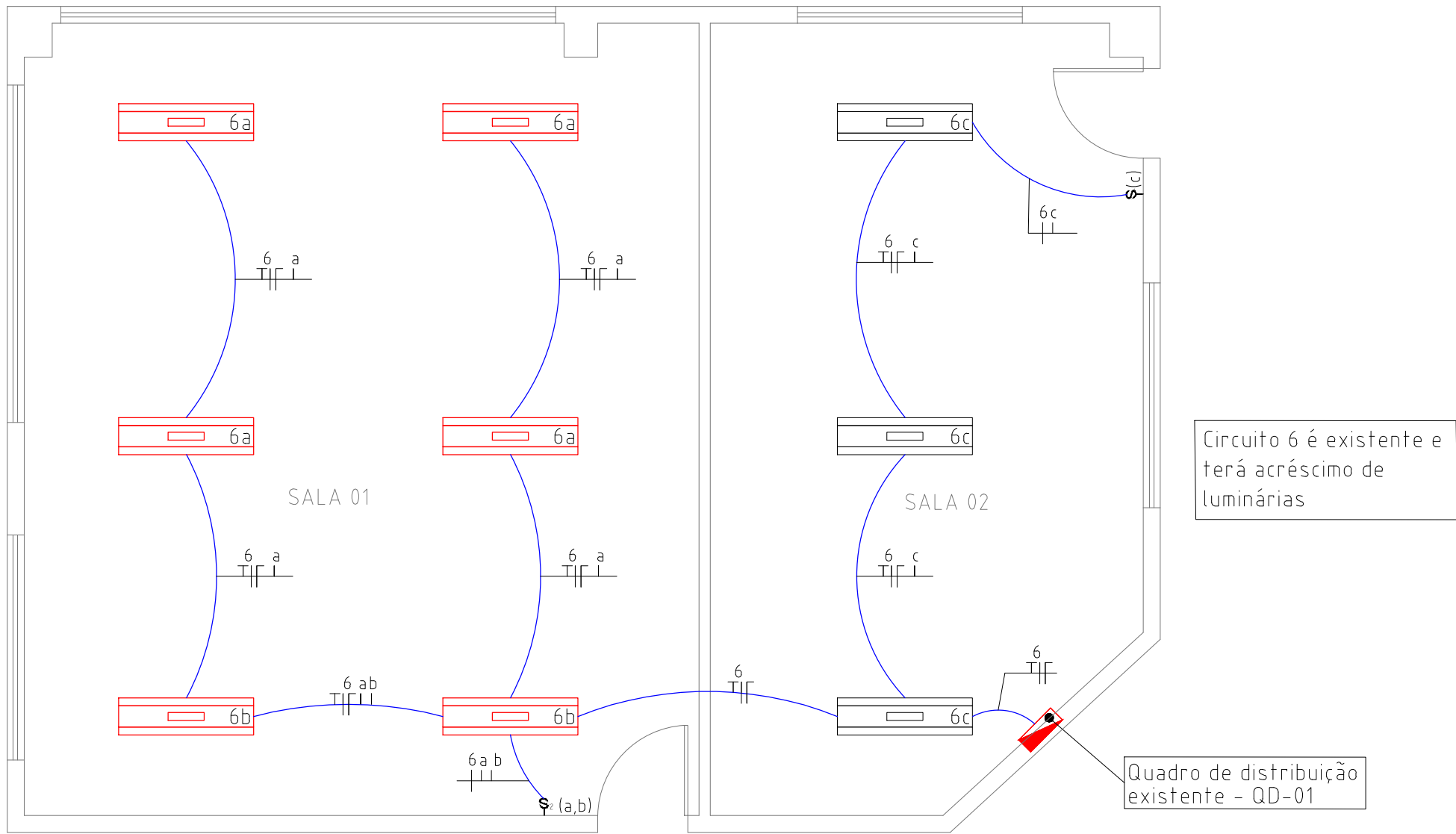
PLANTA BAIXA – ILUMINAÇÃO ESC. 1:50
