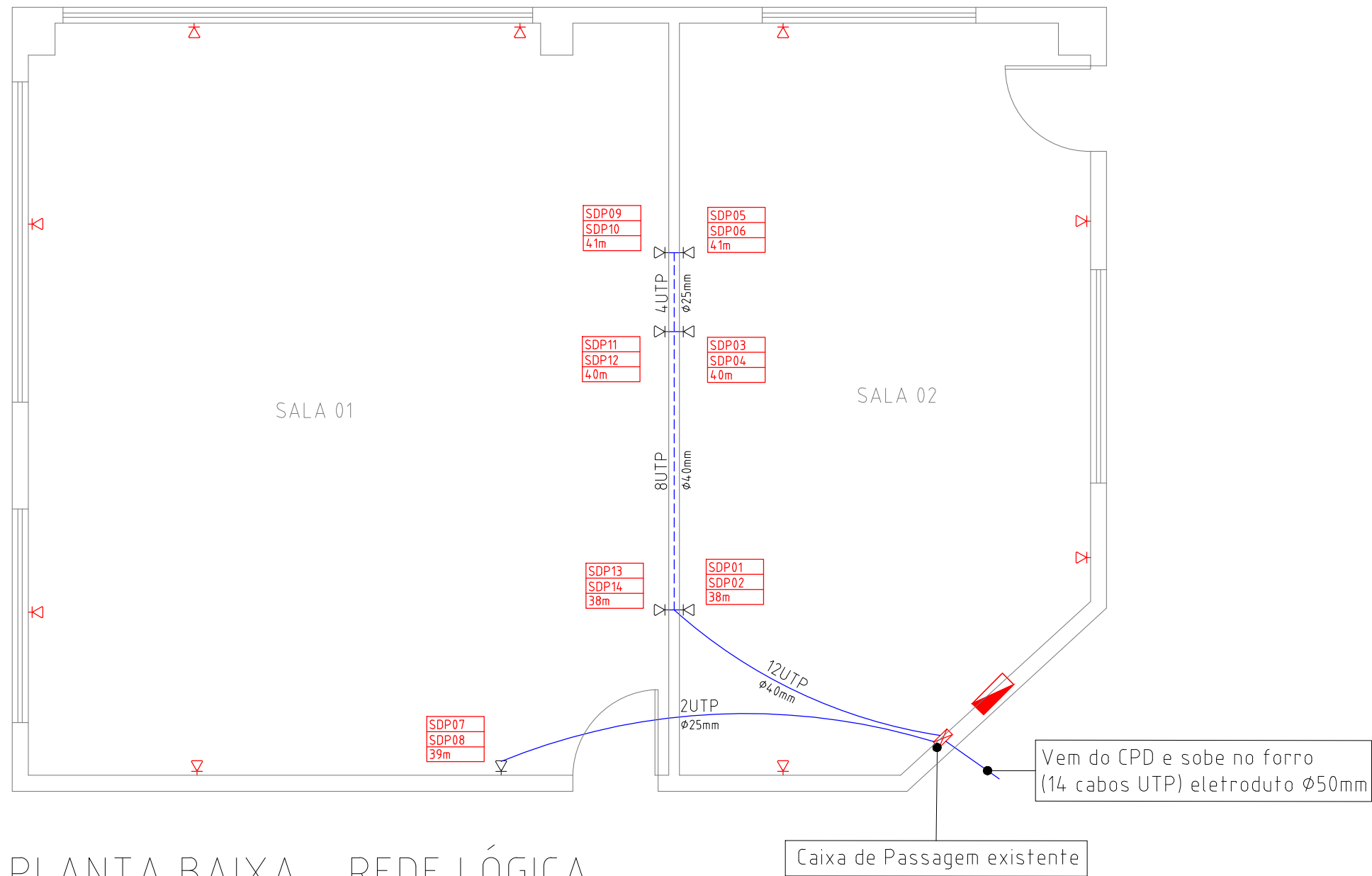
PLANTA BAIXA - REDE LÓGICA ESC. 1:50
