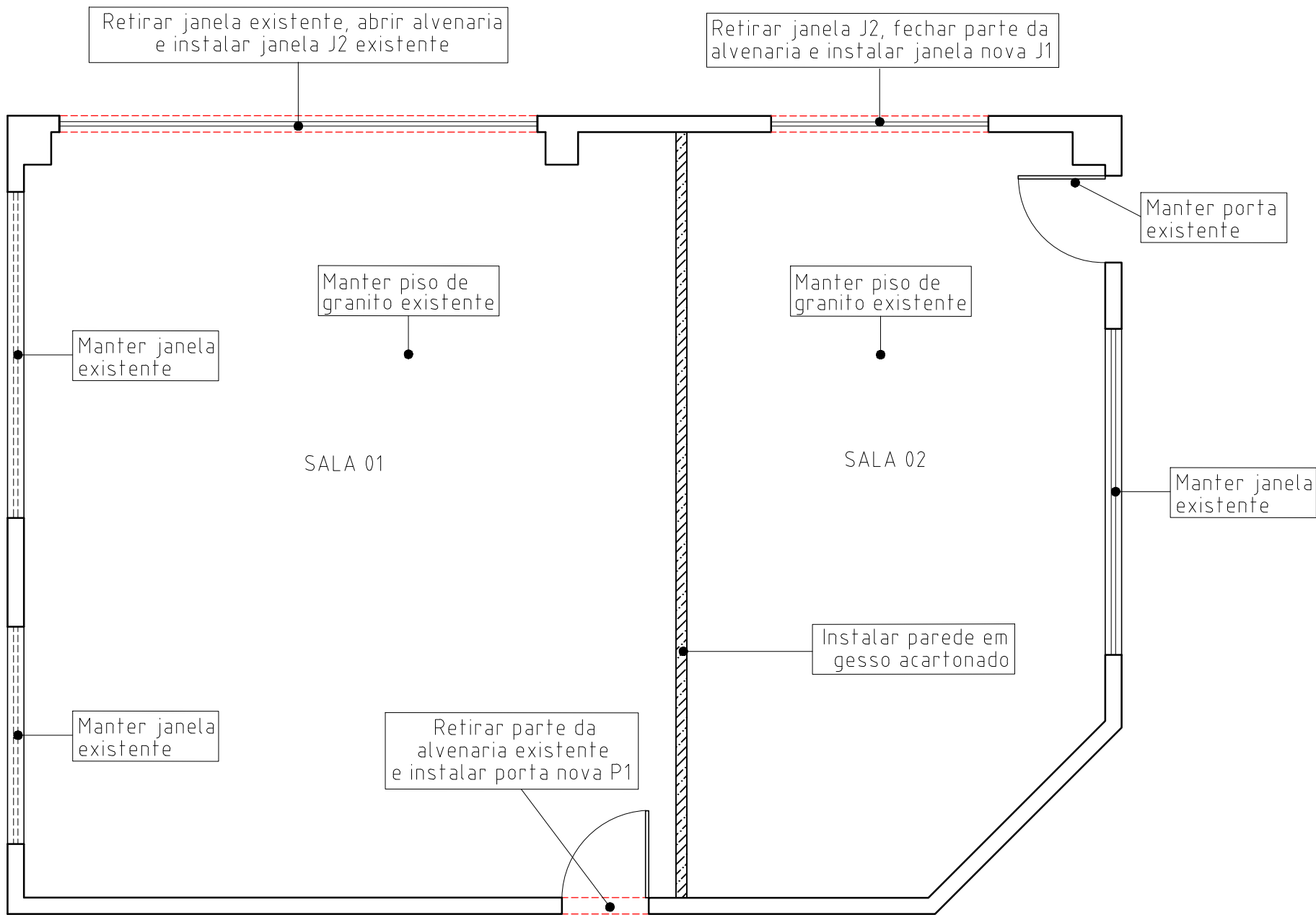
PLANTA BAIXA DE REFORMA ESC. 1:50
